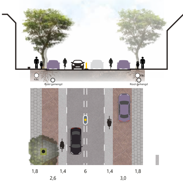
Huidig profiel C
