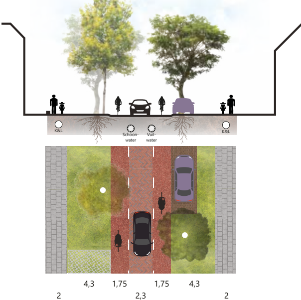
Ontwerp profiel C
