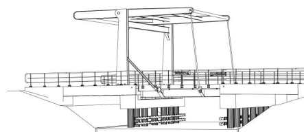
Nieuwe Hallsebrug met bovenbouw.
